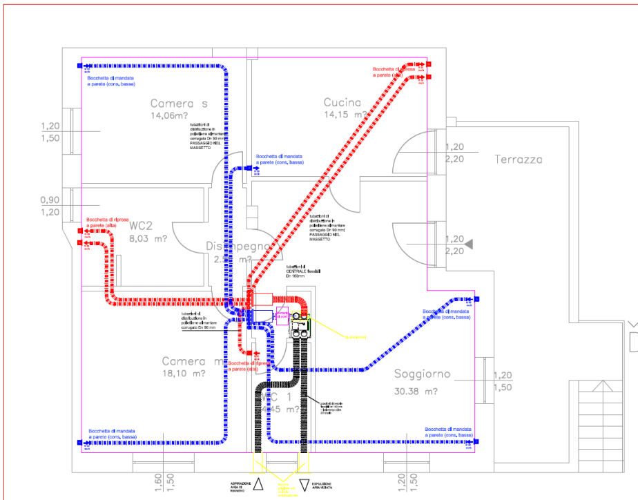
Piante Piano rialzato-stato finale-scala 1.100
