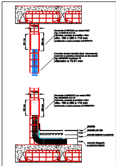
Particolare - posizione bocchette e ingombro tubazioni
