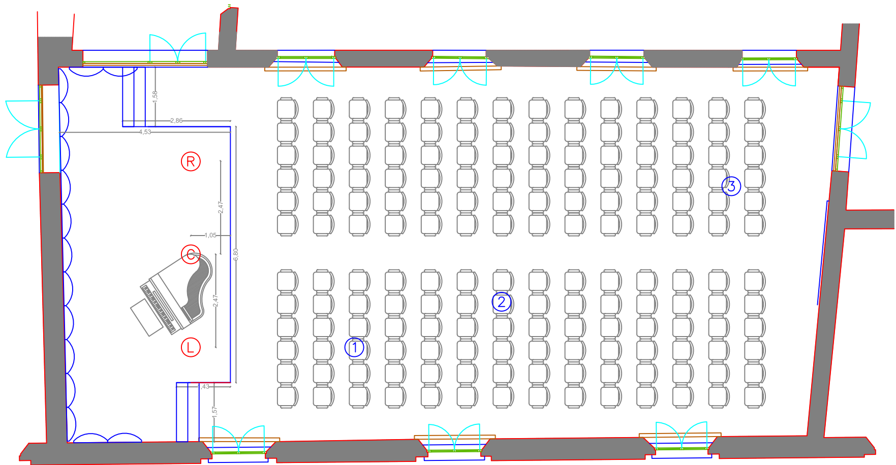
PLANIMETRIA a quota + 2,40 m
